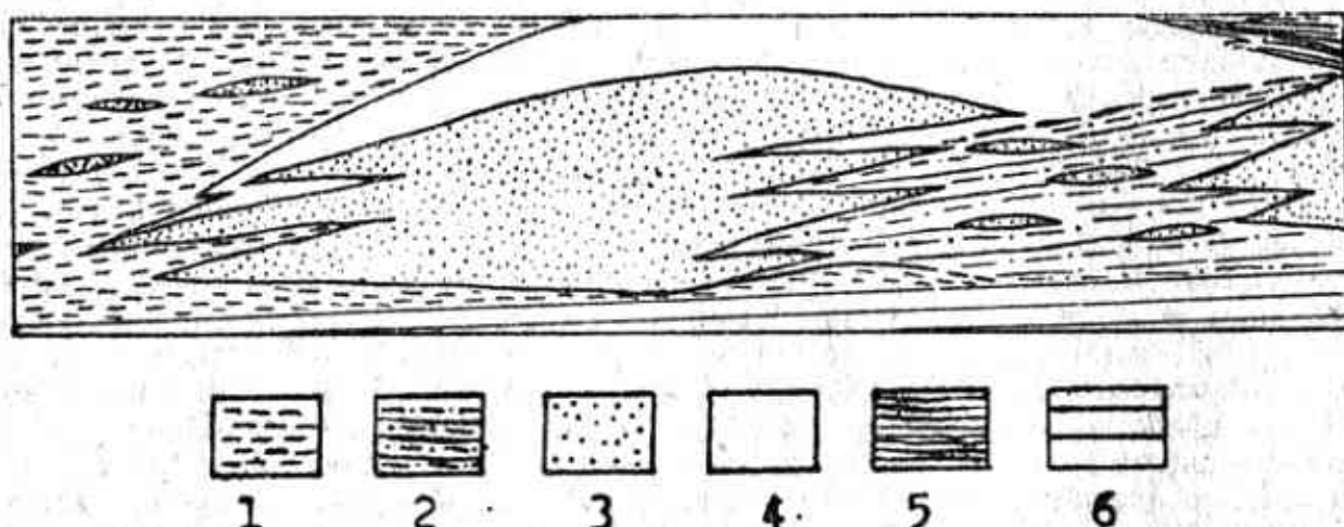
Obr. 2. Schema faciálního vývoje nižší části spodního karbonu v oblasti Šternberka. — Schema der facialen Entwicklung des niederen Teiles des Unterkarbons im Gebiet von Sternberg.
