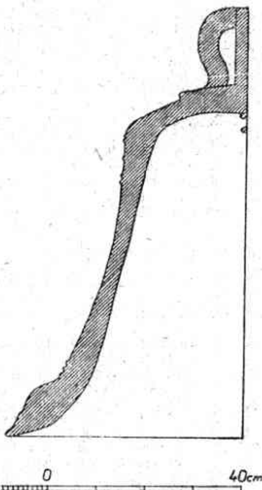
1. Žebro zvonu Zachariáše Milnera z r. 1603 (Podbřežice, okr. Vyškov). Kreslil V. Burian
