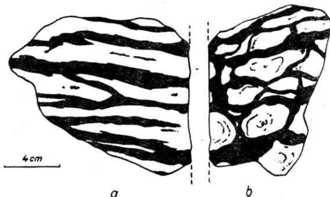
Obr. 3: Rudní agregáty s hlušinou (černě) v přeměněném keratofyrovém popelovém tufu; a — rovnoběžně s lineací, b — kolmo k lineací. Nová jáma, III. patro.
