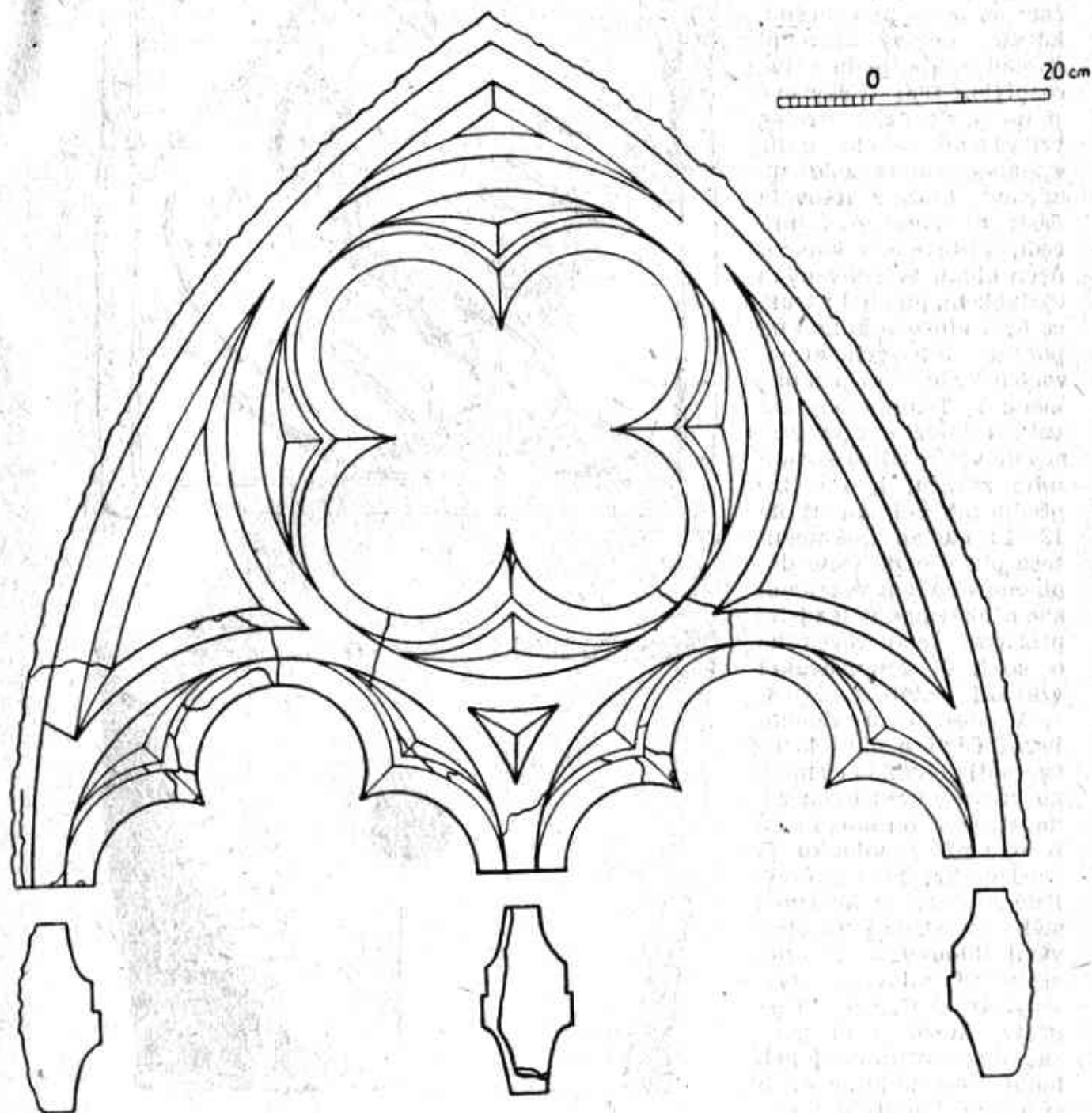
Dolany, Kartouzka: Rekonstrukce okenní kružby kostela.
