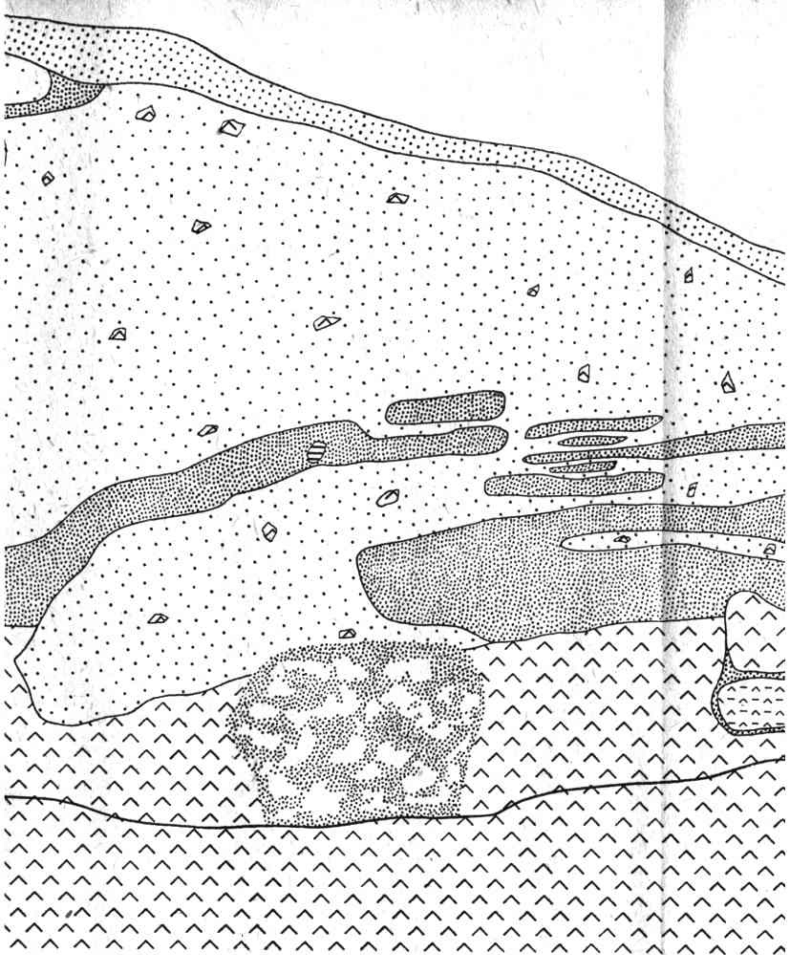
Obr. 2. Profilový řez vnitřním valem na hradisku Podborský, J. Štelcl 1966, kreslil J. 1 — okatá rula, 2 — plagioklasová rula, rula ( p > Kž ), 4 — granát-biotit-muskovitit na s uhlíky, 7 — porušená hlína s uhlíky uhlíků, 9 — písčité polohy, 10 — humus.
