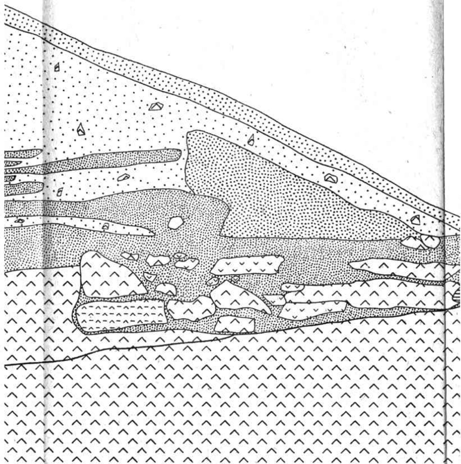
ním valem na hradisku Šance u Plavče. Sestavili V. telci 1966, kreslil J. Palášek. Vysvětlivky značek: — plagioklasová rula, 3 — sillimanit-granát-biotitická granát-biotit-muskovitický svor, 5 — křemen, 6 — hlí- porušená hlína s uhlíky, 8 — hlína s nižším obsahem polohy, 10 — humus.
