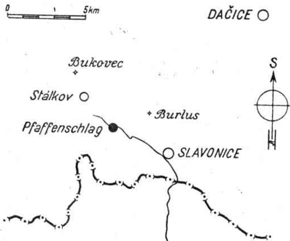
Obr. 3. Schematická geografická situace zaniklé středověké osady Pfaffenschlag u Slavonic.
