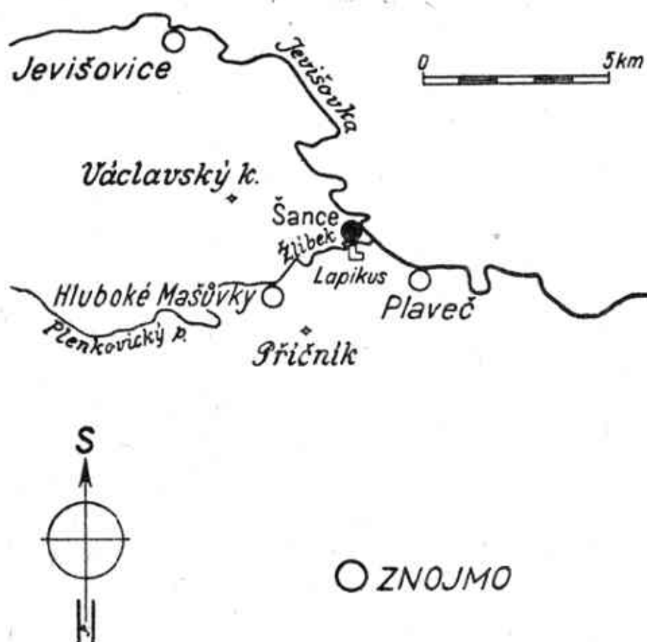
Obr. 1. Schematická geografická situace hradiska Šance u Plavče.
