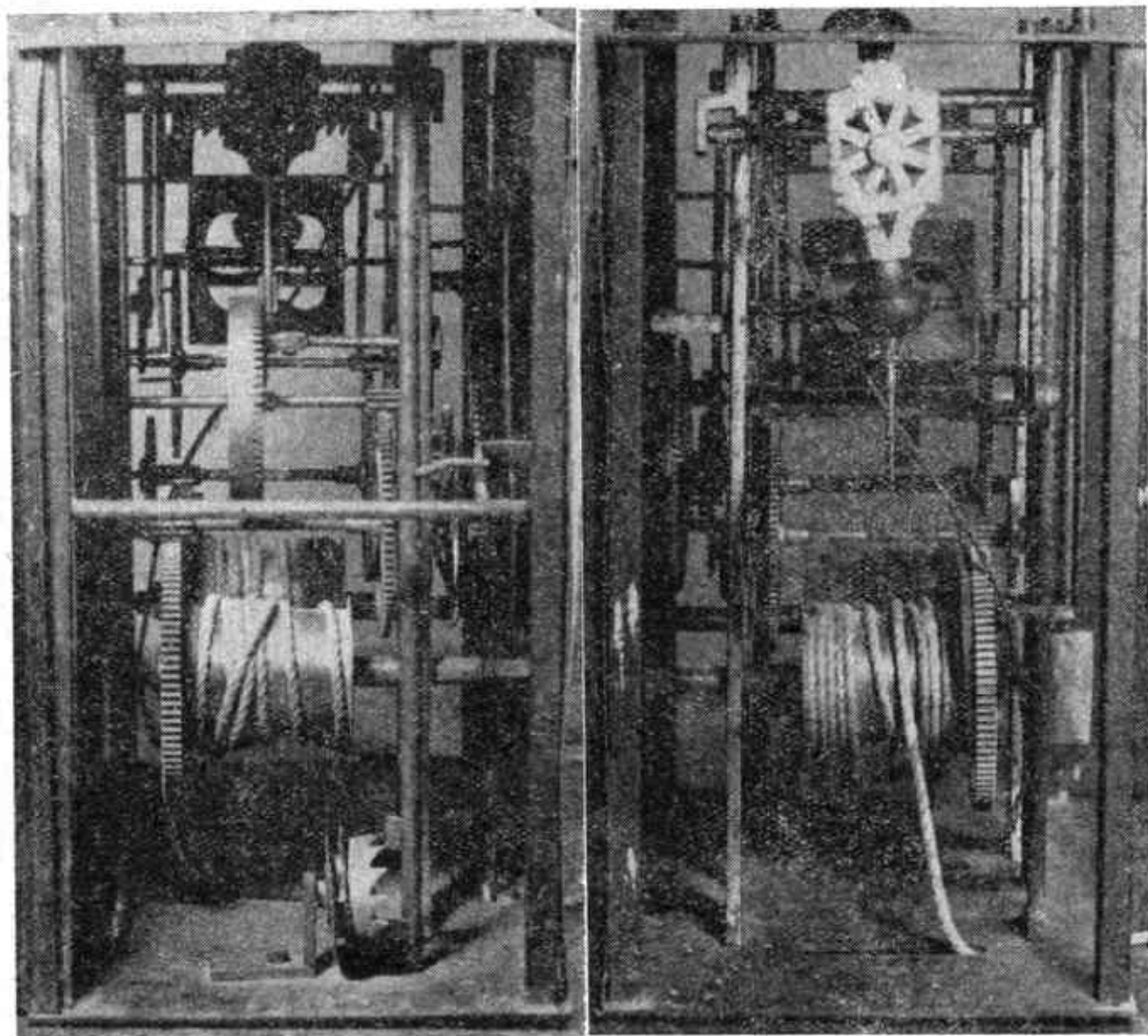
Vnitřek hodinového stroje s vřetenovým krokem.
