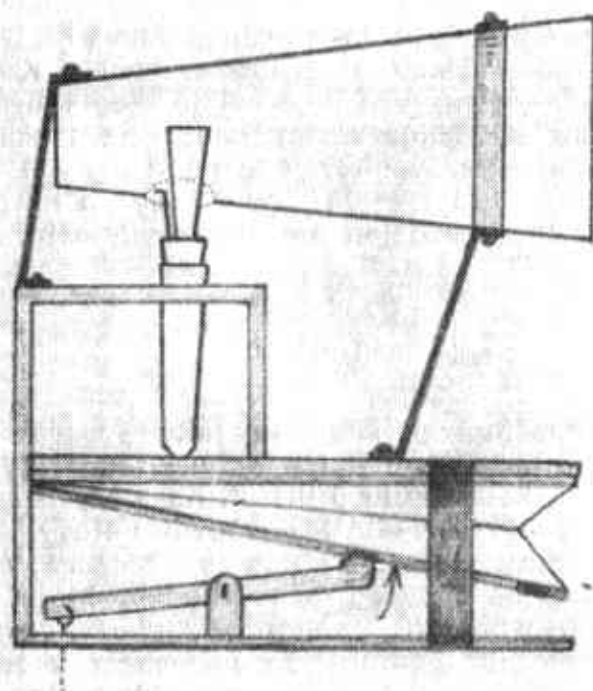
Olomouc, orloj. Mechanismus hlasu kóhouta.
