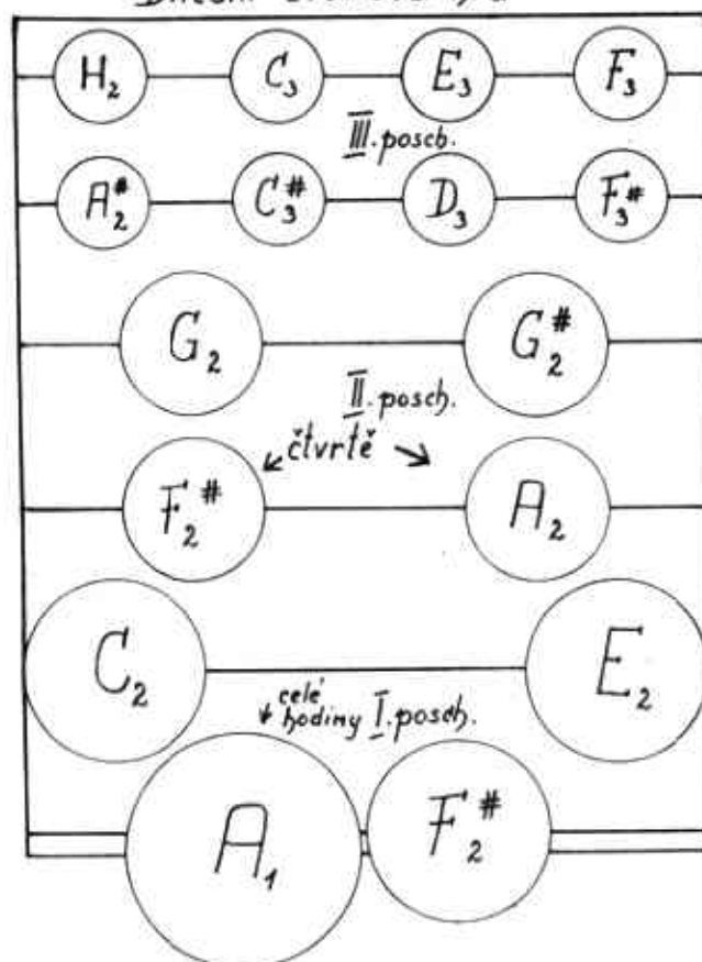
Olomouc, orloj. Schéma rozmístění píšťal a zvonků.
