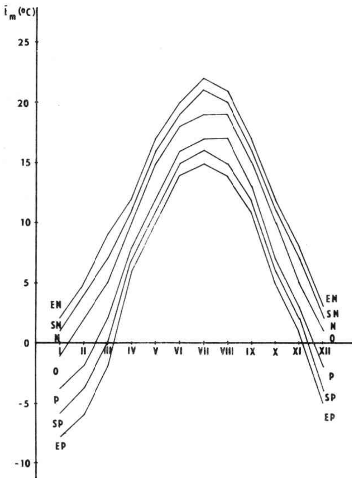
Obr. č. 2: Zóny normality průměrných měsíčních teplot na stanici Tršice (EN — extrémně nadnormální, SN — silně nadnormální, N — nadnormální, O — normální, P — podnormální, SP — silně podnormální, EP — extrémně podnormální)
