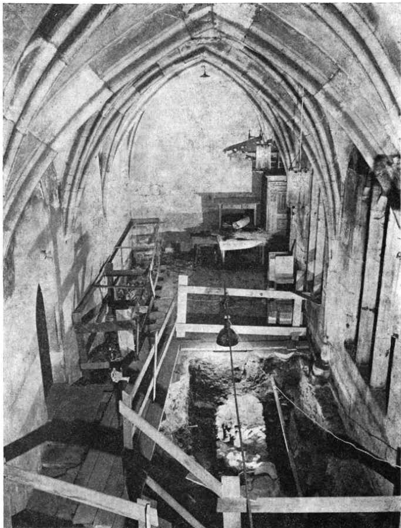
Olomouc, dóm, východní chodba ambitu: Zdivo románského ambitu pod dlažbou ambitu gotického. Foto J. Schubert.
