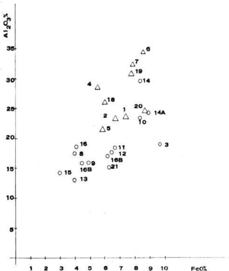
5. Diagram závislosti \text{Al}_2\text{O}_3 na \text{FeO} (korelační koeficient r = 0,66 ).
