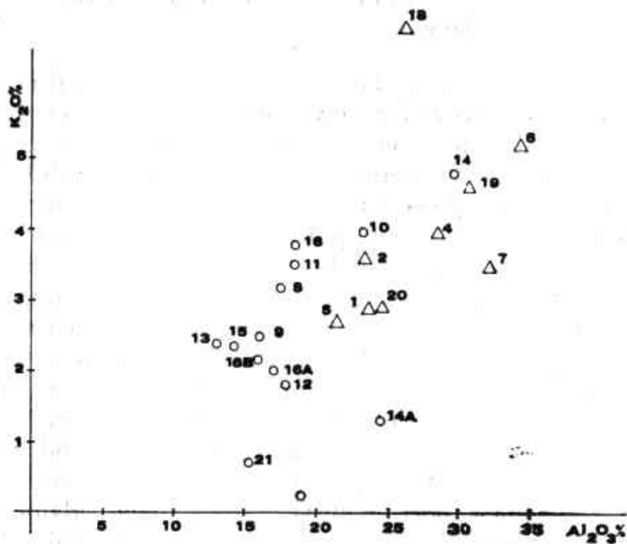
11. Diagram závislosti K_2O na Al_2O_3 (korelační koeficient r = 0,66 )
