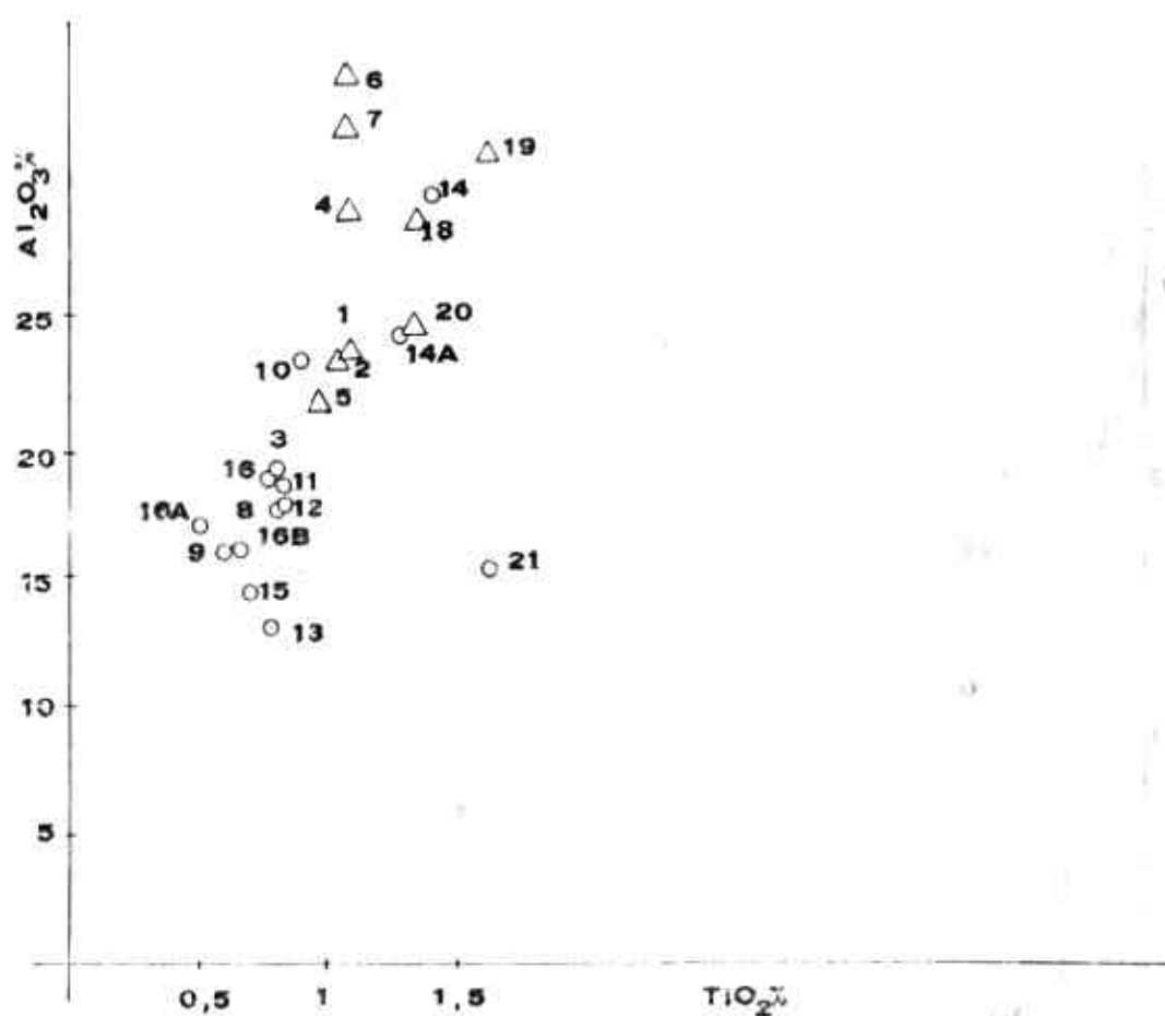
4. Diagram závislosti \text{Al}_2\text{O}_3 na \text{TiO}_2 (korelační koeficient r = -0,65 )
