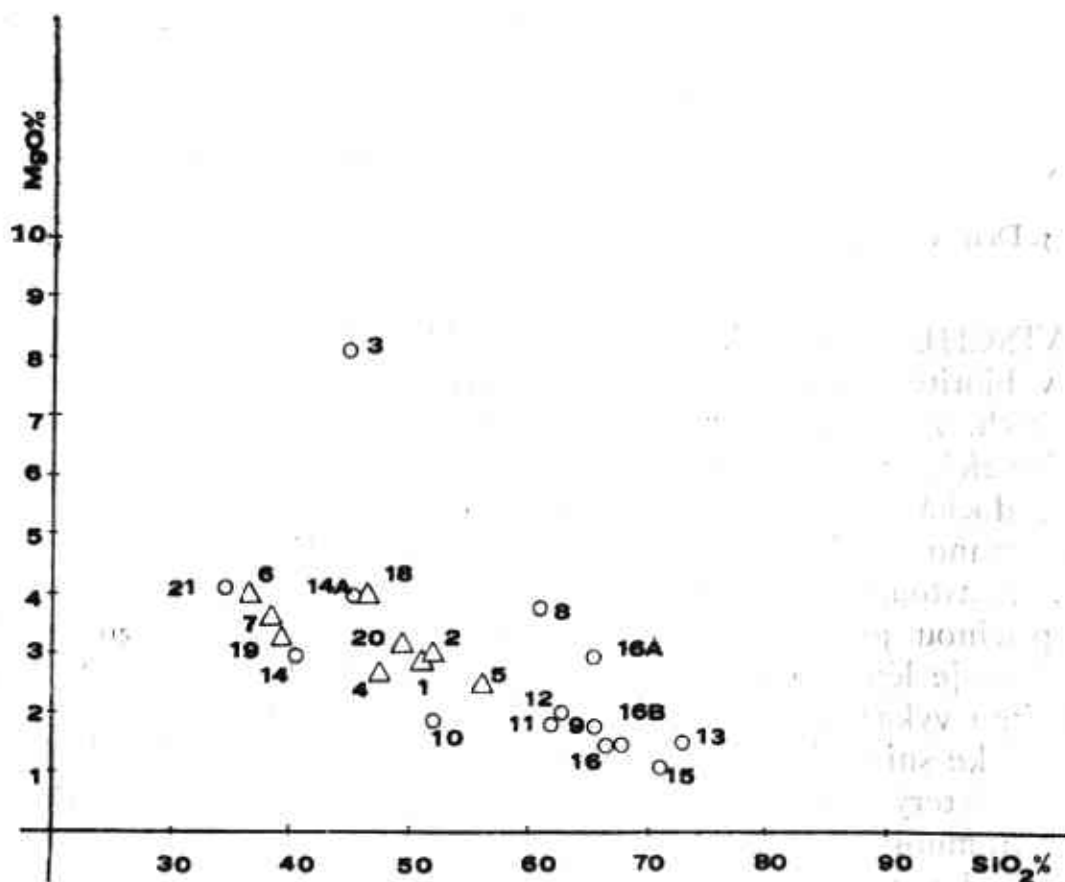
7. Diagram závislosti MgO na \text{SiO}_2 (korelační koeficient r = -0,83 )
