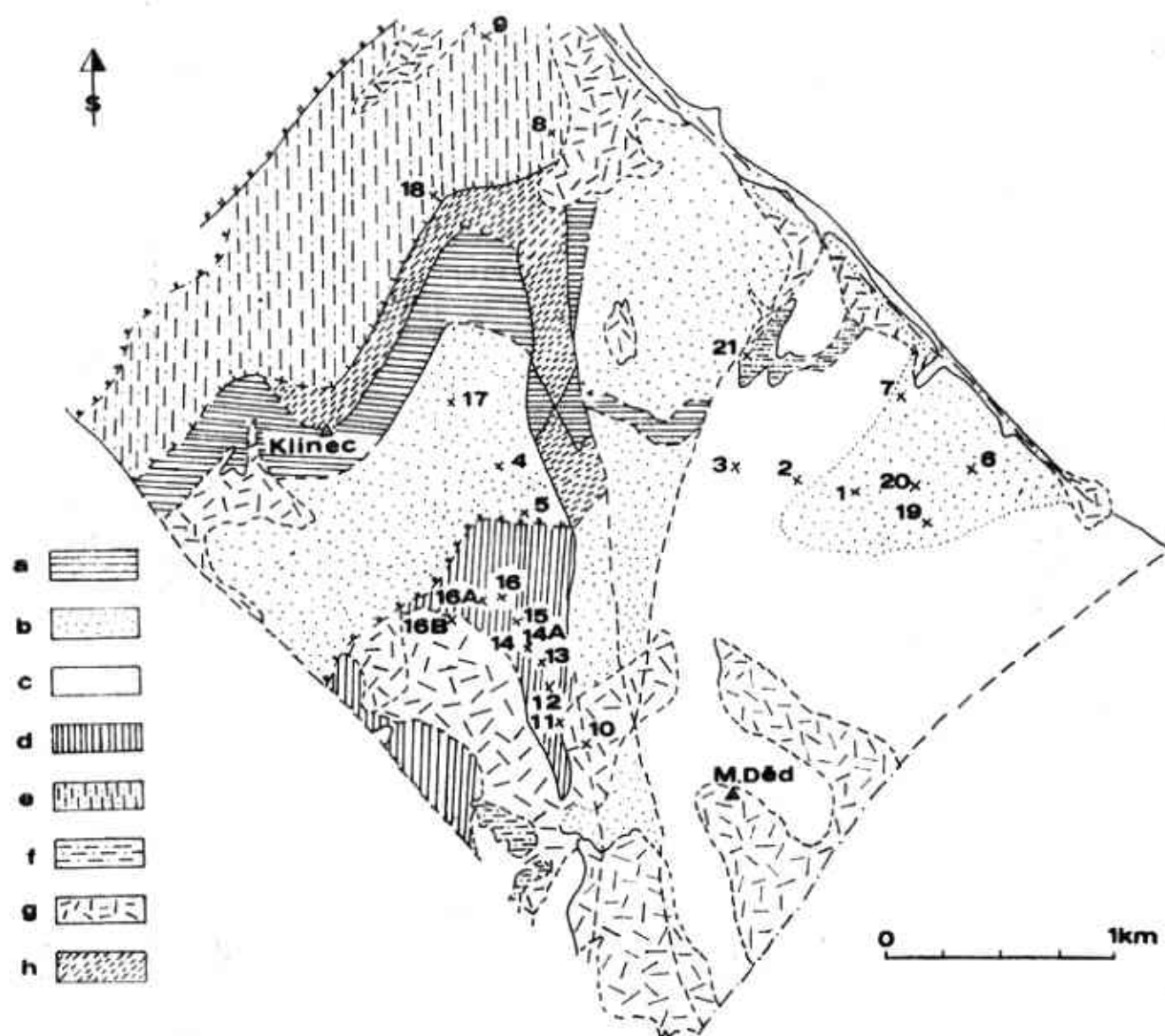
1. Schématická mapka části desenské jednotky s vyznačením míst odběru vzorků: a) – amfibolit, b) – plagioklasový fylit, c) – chlorit-muskovitický fylit, d) – páskovaná retrográdně metamorfovaná rula, e) – muskovit-chloritická rula, f) – zelená břidlice, g) – deluviální sedimenty, h) – porfyroid.
