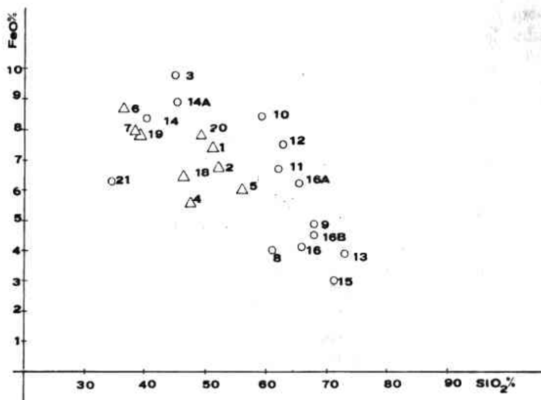
6. Diagram závislosti FeO na \text{SiO}_2 (korelační koeficient r = -0,72 )
