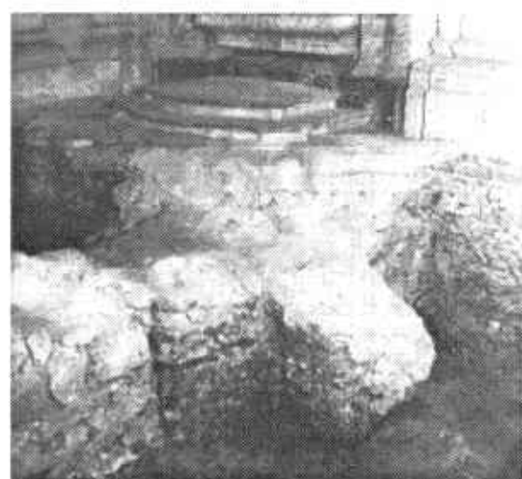
Abb. 8. Fundament 17 der Südstütze des Lettnerpodiums. Rechts und links von einer Fuge getrennt die Mauern 16 und 18 der Vorhalle. Blick von Nordwesten.
