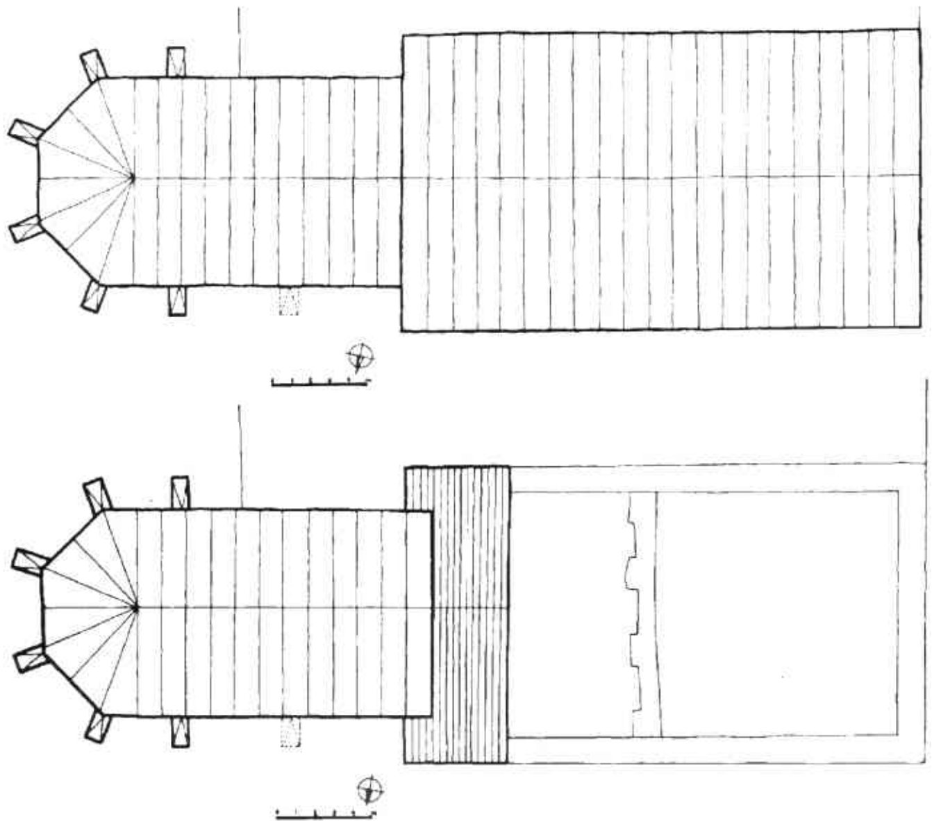
Abb. 16. Kirche der hl. Kreuzerhöhung. Blick aus der Vogelperspektive auf den gotischen Bau vor und nach dem Abriss des Kirchenschiffes, an dessen Stelle eine vor den Chorgebaute niedrigere Vorhalle trat.
