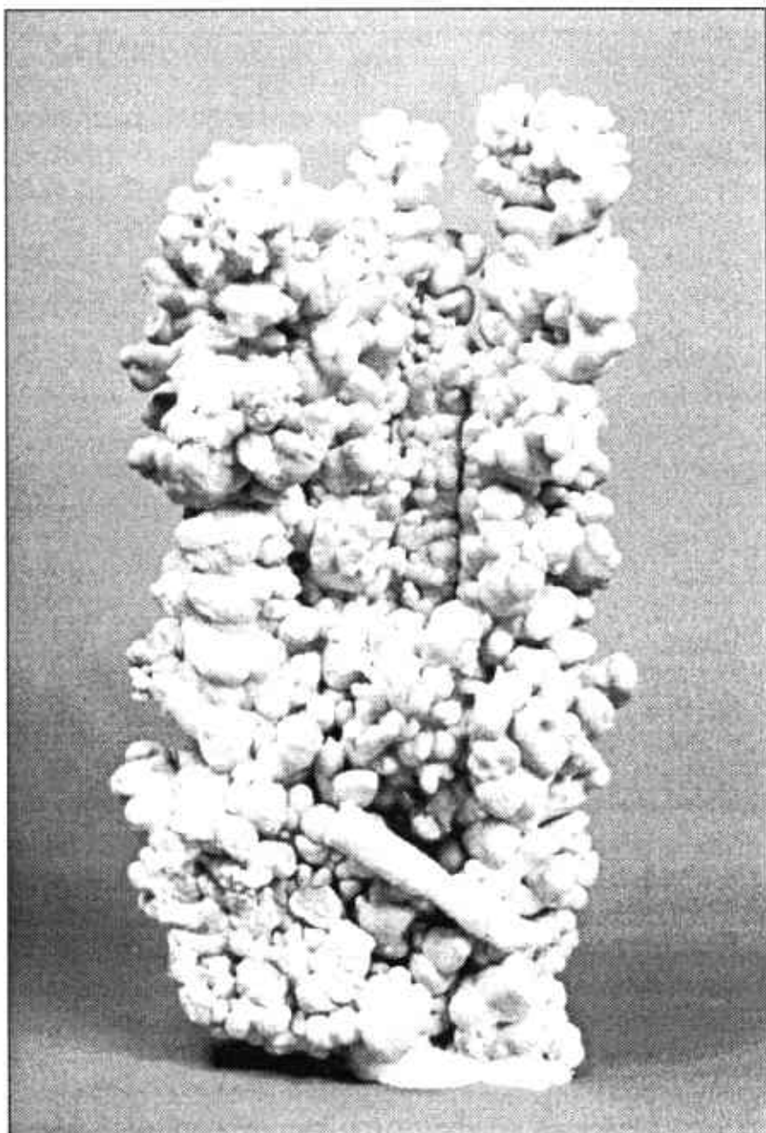
Vzorek sintrových anomálií - pisolitů - hlavního typu výplní puklinových jeskyní ve Vitošově.
