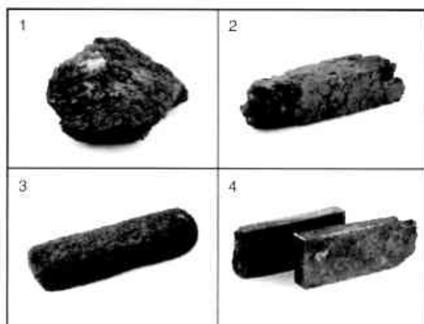
Obr. 1 Vytavená lupa přímo z pece ve tvaru velké houby. Obr. 2 Zpracovávaná lupa kovářím a postupným stmelováním za teploty cca 1200 °C. Obr. 3 Litím odpíchnutá ocel ve tvaru hřívny přímo z pece. Obr. 4 Malé bloky oceli vzniklé překládáním a kovářím. Foto archiv autora.
