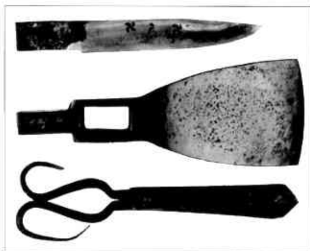
Příklad nástrojů denní potřeby s navařovanou břitovou ocelí. U nože v horní části je patrná kalená linie břitu a struktura překládů. Foto archiv autora.
