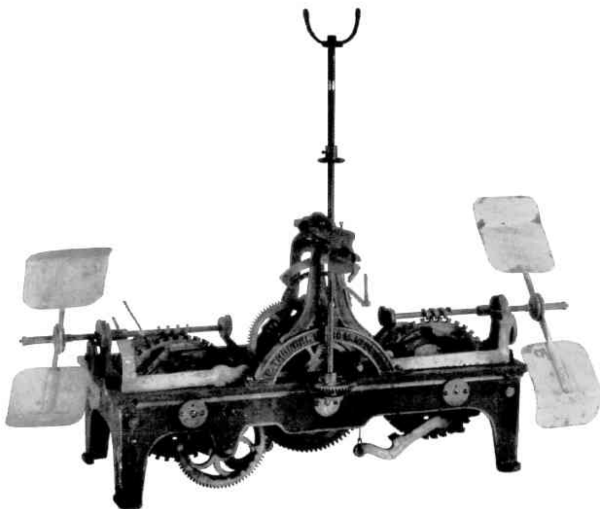
Stroj věžních hodin, R. Thöndel, Uničov, 1919 (Foto: P. Rozsival)
