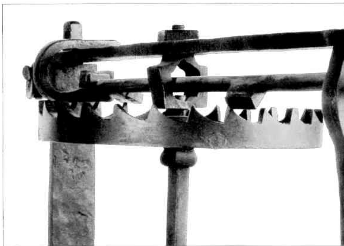
Detail vřetenového kroku (korunové kolo s paletovým hřídelem) stroje věžních hodin, M. Vogt, Olomouc, 1737. (Foto: P. Rozsival)
