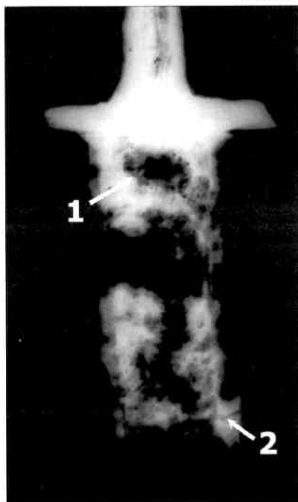
Rentgenový snímek hlavice meče: 1 – část vkovaného damaškového drátu, 2 – zásek v čepeli meče (Vojenská nemocnice Hradisko)
