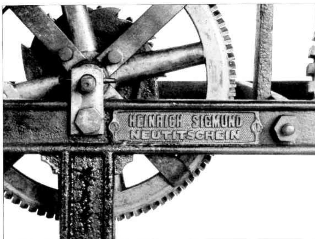
Detail signatury výrobce stroje věžních hodin: HEINRICH SIGMUND NEUTITSCHEN, Nový Jičín, přelom 19. a 20. století (Foto: P. Rozsival)
