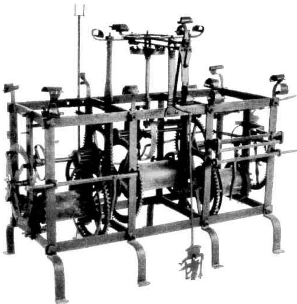
Stroj věžních hodin, F. Lang, Uherské Hradiště, 1734 (Foto: P. Rozsival)
