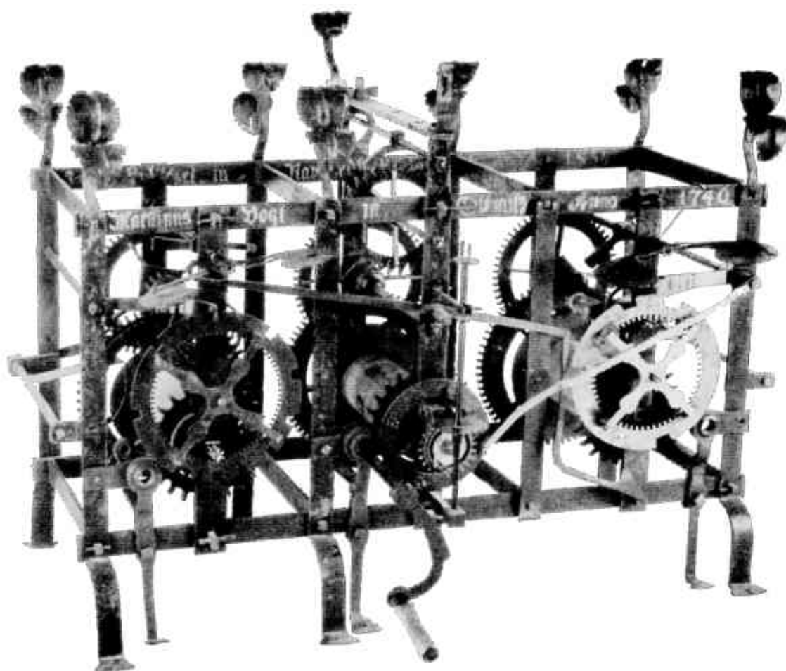
Stroj věžních hodin z kostela v Pohořelicích na Zlínsku, M. Vogt, Olomouc, 1740, renovoval J. Kubíček, Napajedla, 1834 (Foto: P. Rozsival)
