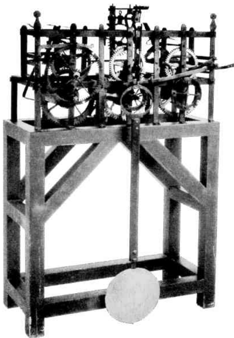
Stroj věžních hodin na dřevěném podstavci, Plzeň, přelom 18. a 19. století (Foto: P. Rozsival)
