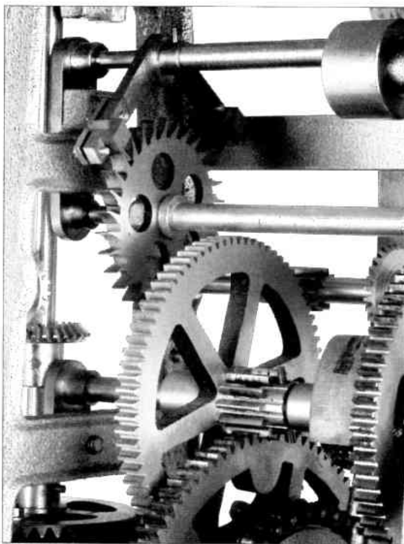
Detail Grahamova kotvového kroku na věžním hodinovém stroji, OPP Vyškov, 80. léta 20. století (Foto: P. Rozsívál)
