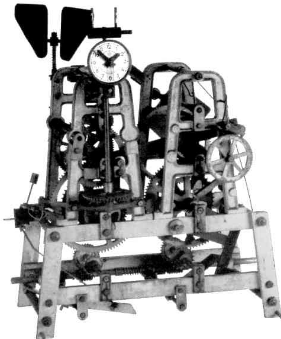
Věžní hodinový stroj z Nové radnice v Ostravě, OPP Vyškov, 70. léta 20. století (Foto: P. Rozsival)
