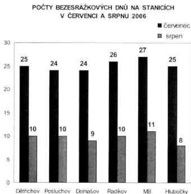
Obr. 5 Počty bezsrážkových dnů na stanicích v červenci a srpnu Fig. 5 Number of days without precipitation in July and August
