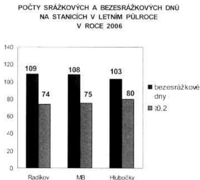
Obr. 4 Srážkové a bezsrážkové dny na stanicích v letním půlroce Fig. 4 Number of days with and without precipitation in the warm half-year
