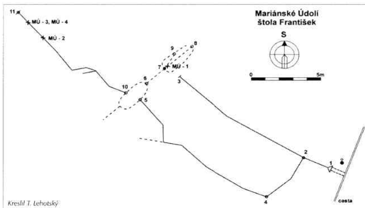
Obr. 1. Schéma štol František s místy odběru vzorků MÚ-1, MÚ-2, MÚ-3, MÚ-4
