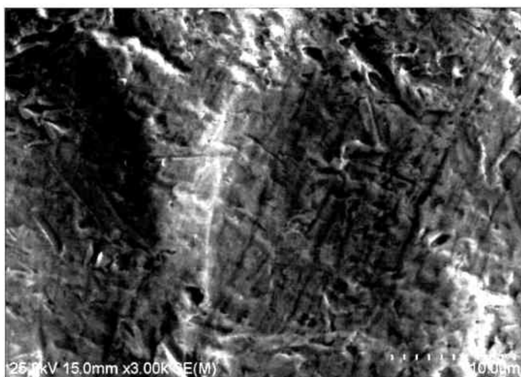
Obr. 2. Zonální stavba zlatinky vyrýžované z potoka Zlatý důl.
