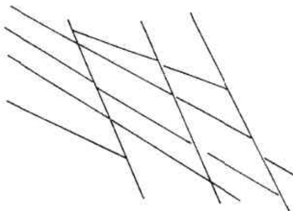
Obr. 2: Kamenolom Šternberk – Horní Žleb Schematické vyjádření systému příčných puklin s dvojitou velikostí sklonu. Situace velmi častého vývoje puklinatosti v různých úsecích těžbou odkrytých stěn mezi jednotlivými etážemi lomu.
