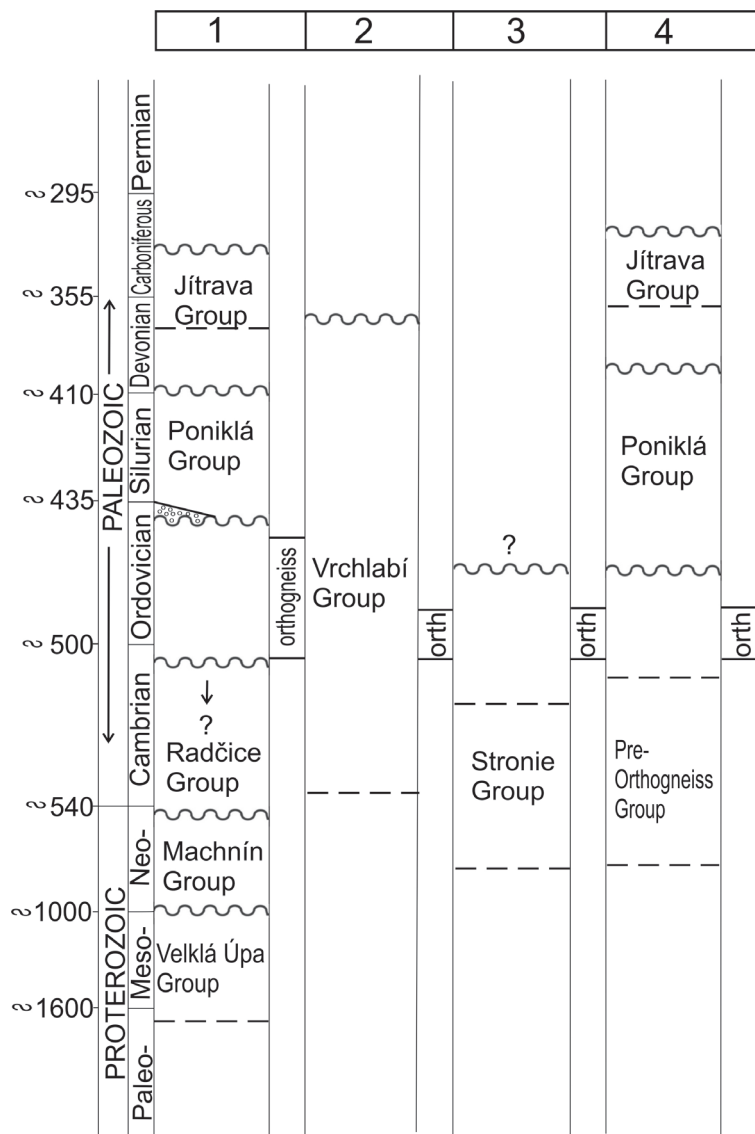
Obr. 1. Korelační schéma jednotek
