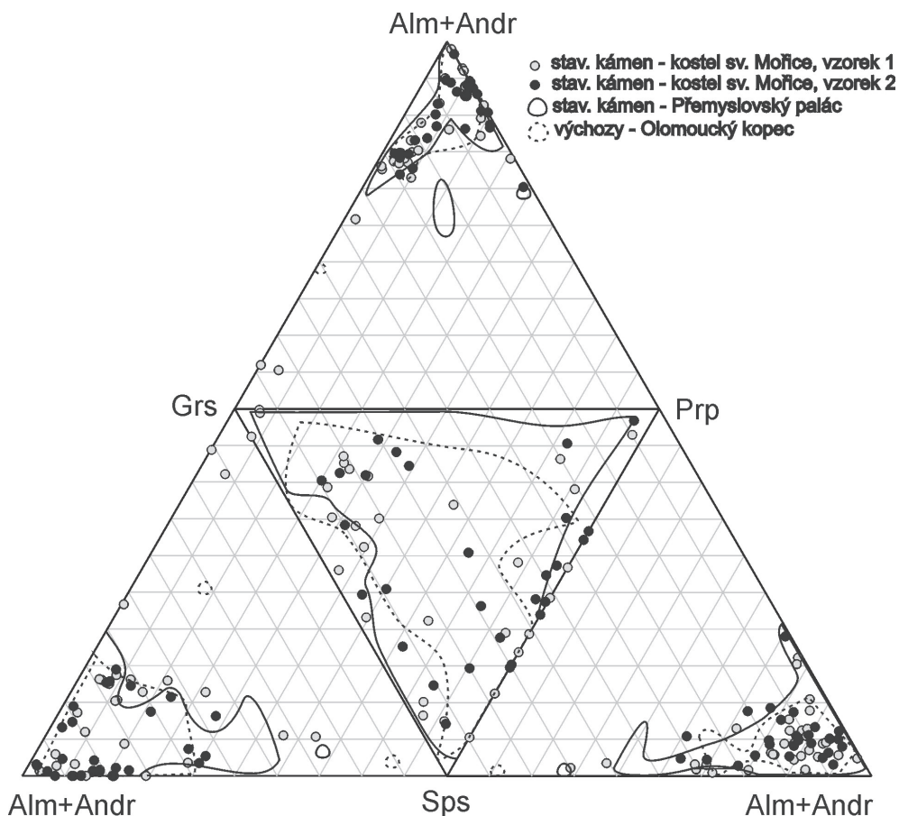
Obr. 4. Grafické znázornění chemismu detritických granátů. Srovnávací data (droby ze stavby Přemyslovského paláce a droby z výchozů na Olomouckém kopci) jsou z práce ČOPIJKOVÉ et al. (2007).
