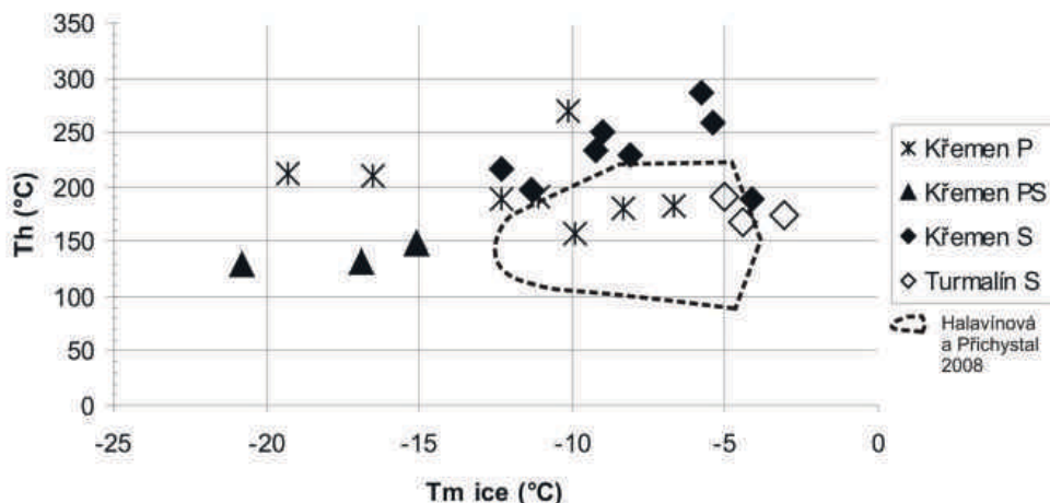
Obr. 1. Diagram pro Th/Tm ice dvoufázové L+V inkluze vodných roztoků (Th = teplota homogenizace, Tm ice = teplota tání posledního ledu, L = kapalina, V = plyn)
