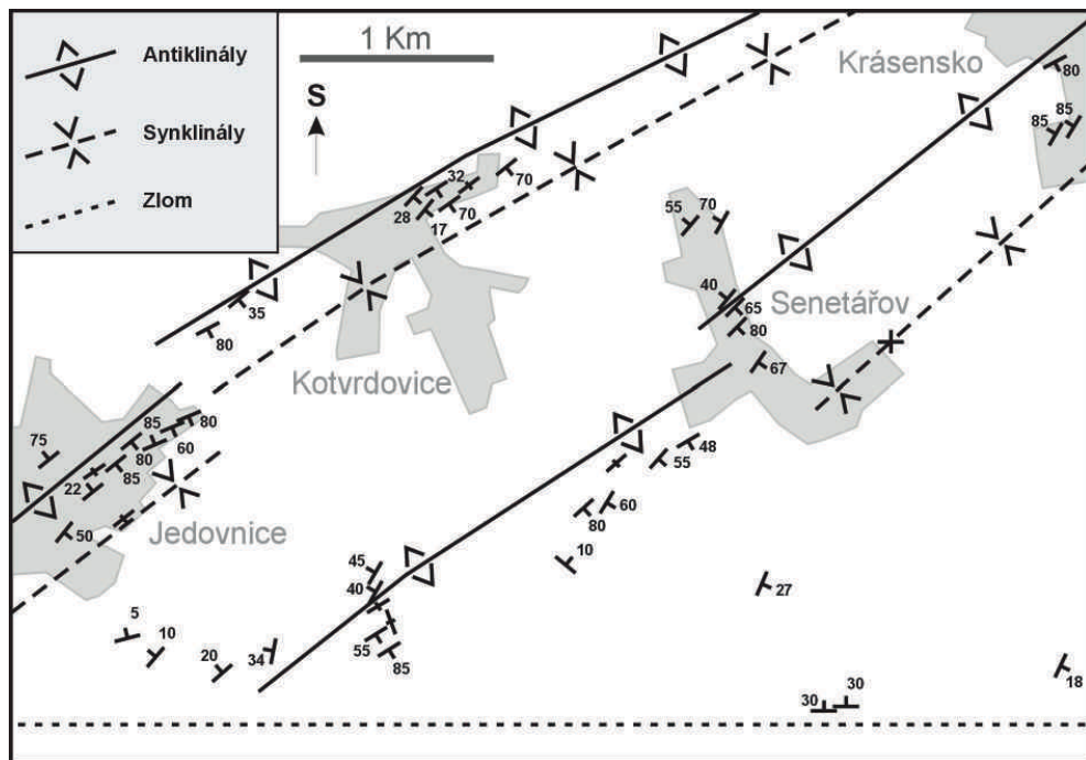
Obr. 2. Schematická strukturní mapa severovýchodního okraje listu Jedovnice 24–411 s vyznačenými orientacemi vrstevnatosti a průběhy stop osních ploch v kulmských sedimentech.
