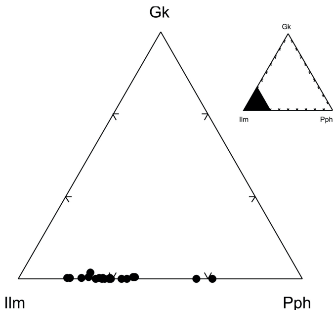
Obr. 1. Chemické složení ilmenitu. Fig. 1. Chemical composition of ilmenite.
