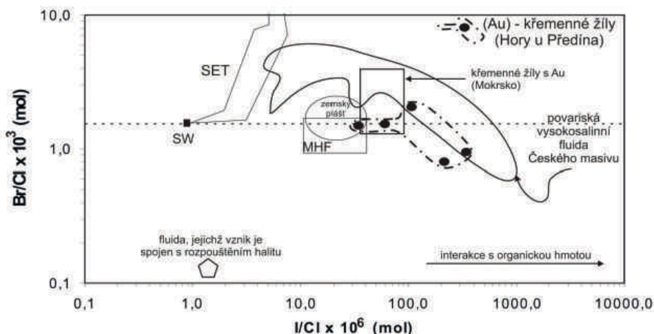
Obr. 2. Diagram I/Cl vs. Br/Cl výluhů fluidních inkluzí z Hor u Předína a jejich srovnání s fluidy různého původu. Převzato a upraveno podle DOLNÍČKA et al. (2009). SW mořská voda, SET linie evaporace mořské vody, MHF nekontaminovaná magmatická hydrotermální fluida.
