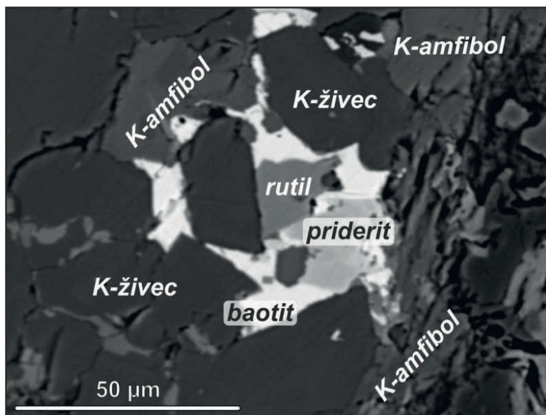
Obr. 3. Příklad zatlačování intersticiálního baotitu mladší minerální asociací s prideritem a rutilem (snímek ve zpětně odražených elektronech).
