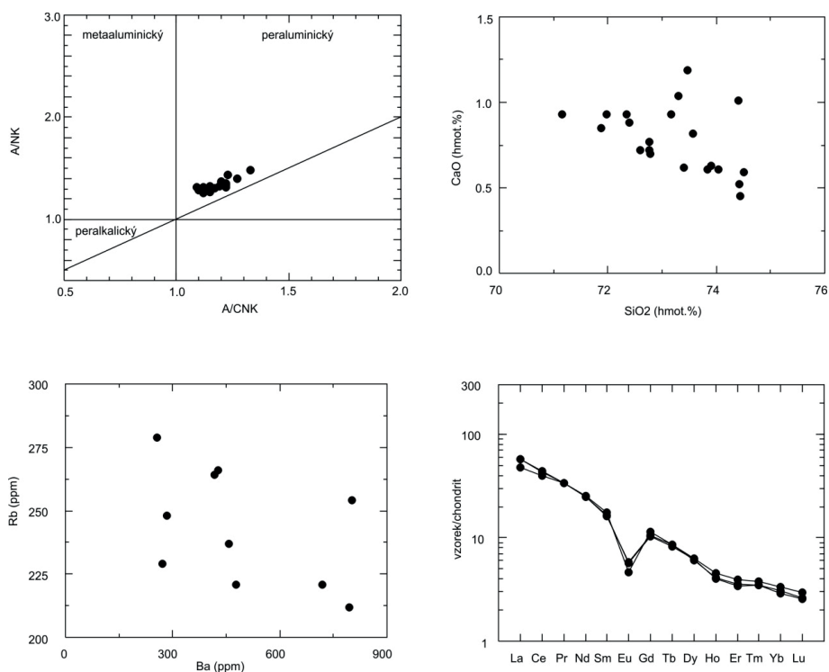
Obr. 3. Chemické složení granitů.
