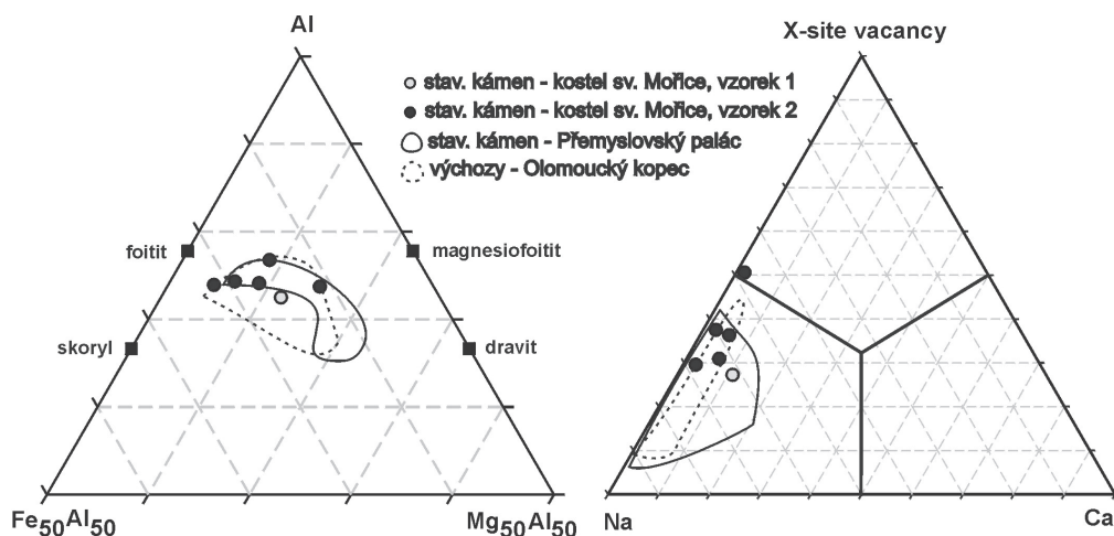
Obr. 5. Chemické složení detritických turmalínů. a – diagram Fe-Mg-Al, b – diagram Na-Ca-vakance v X-pozici. Srovnávací data (droby ze stavby Přemyslovského paláce a droby z výchozů na Olomouckém kopci) jsou z práce ČOPIJKOVÉ et al. (2007).
