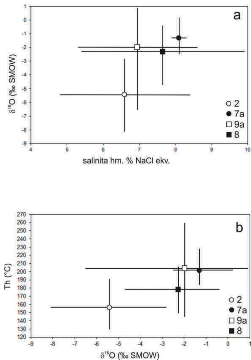
Obr. 1. a – Graf závislosti \delta^{18}\text{O} fluid na salinitě primárních fluidních inkluzí. b – Graf závislosti \delta^{18}\text{O} fluid na Th primárních fluidních inkluzí. Čarami jsou v grafu vyznačeny rozsahy hodnot pro daný vzorek, bodovou značkou jsou vyneseny průměrné hodnoty. 2 – Štůlně; 7a – Zákopy; 9a – Zákopy; 8 – Malý Štítek.
