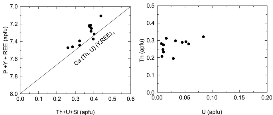
Obr. 2. Chemické složení monazitu.
