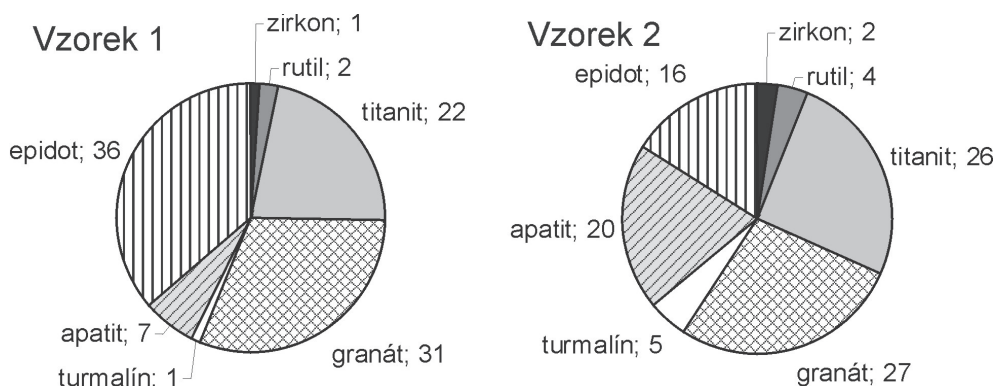
Obr. 3. Koláčové diagramy výskytu těžkých minerálů ve vzorcích drob č. 1 a 2 z kostela sv. Mořice. Číselné hodnoty u každé položky indikují procentické zastoupení.
