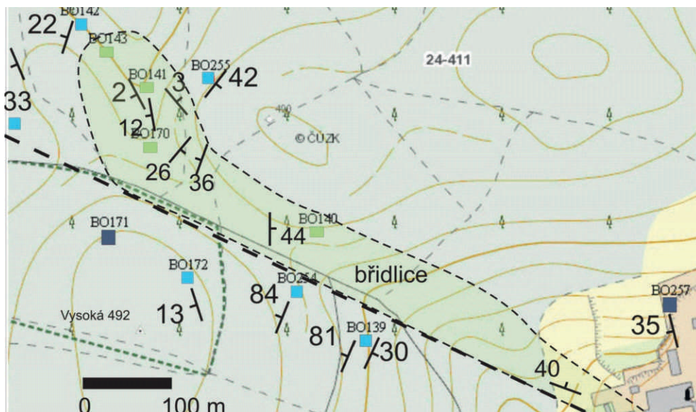
Obr. 2. Schéma znázorňující uložení březinských břidlic do paleokrasového povrchu vápenců (a) a společné provrásnění během variské orogeneze (b).
