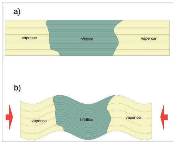
Obr. 1. Strukturní a geomorfologická situace západně od Březiny. Břidlice viséského stáří (uvnitř přerušované čáry) jsou zcela obklopeny devonskými vápenci.
