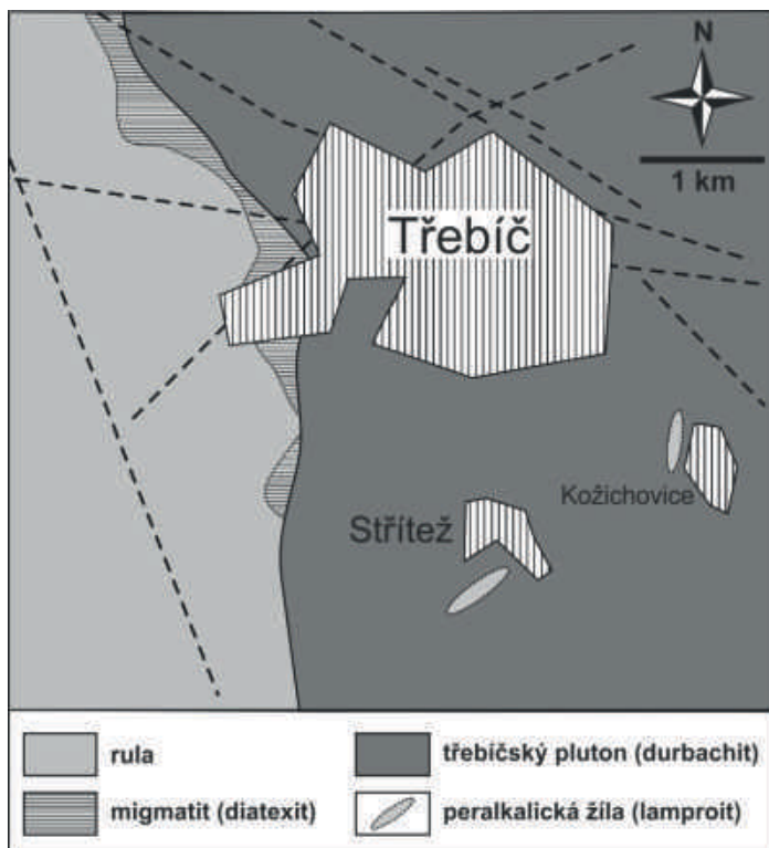
Obr. 1. Pozice výskytů peralkalických žil v třebíčském plutonu. Velikost žil byla kvůli přehlednosti nadhodnocena. Fig. 1. Occurrences of peralkaline dykes in the Třebíč Pluton. The size of the dykes were overestimated for clarity.
