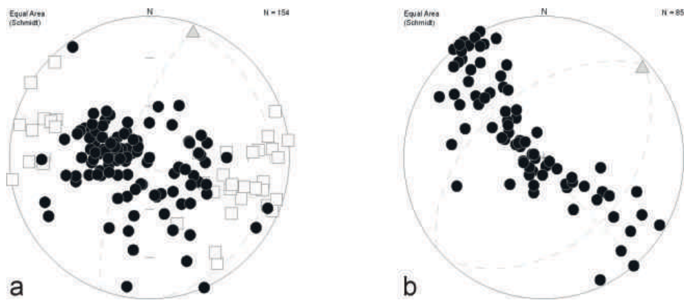
Obr. 1. Orientace vrstevnatostí (plné kroužky) a klivází (prázdné čtverečky) ve vápencích (a) a v kulmských horninách (b) na listu Jedovnice 24–411. Šedé trojúhelníky vyjadřují orientaci osy stavby. Lambertova rovnoplochá projekce na spodní polokouli.
