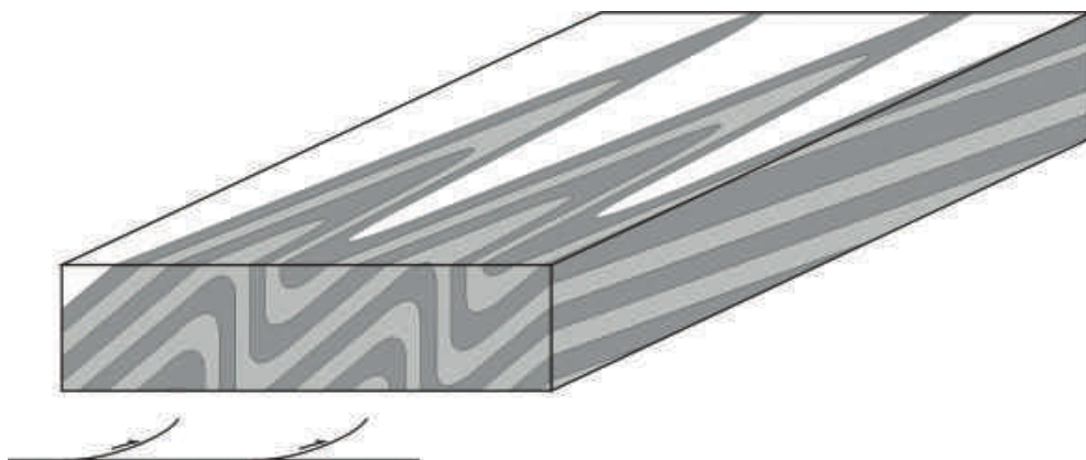
Obr. 3. Blokdiagram nastiňující tektonickou stavbu v kulmských sedimentech. Osa vrás je ukloněna pod úhlem asi 3° směrem k SV. Šířka blokdiagramu cca 2,5 km.
