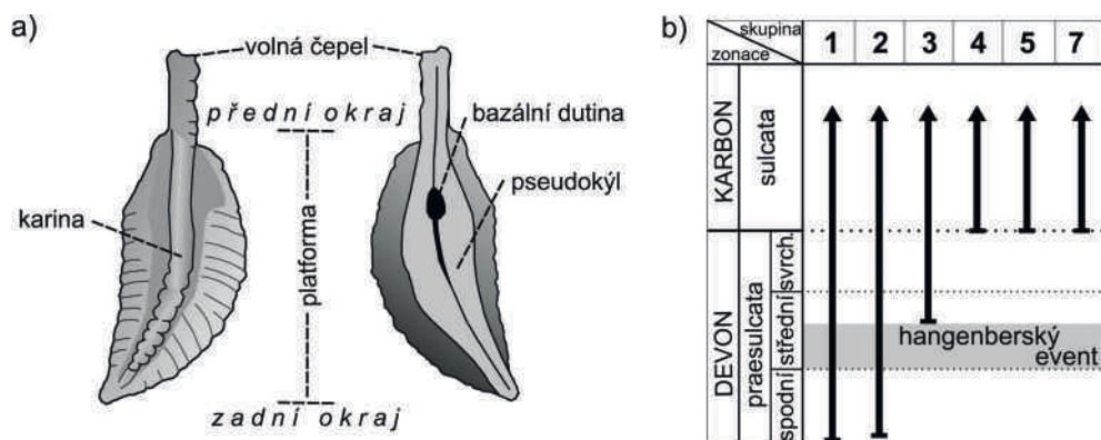
Obr. 1. (a) Klíčové znaky pro klasifikaci platformních elementů rodu Siphonodella . (b) První výskyty morfotypových skupin nejstarších zástupců rodu Siphonodella z jižní a střední části Moravského krasu.
